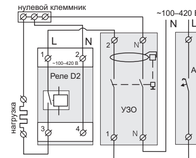
Схема 2. Подключение автоматического выключателя и УЗО без транзита нуля через реле
